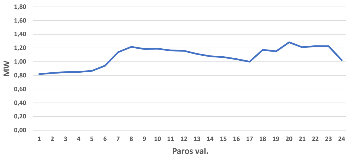
Paros vidutinis šilumos poreikio grafikas nešildymo sezono metu Pasvalyje
