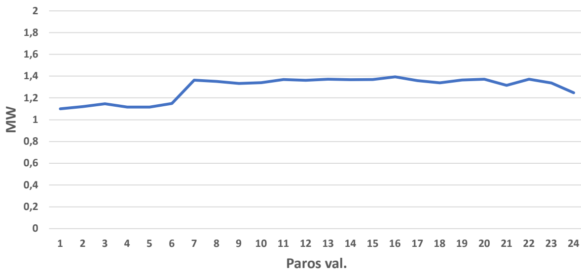
Paros vidutinis šilumos poreikio grafikas nešildymo sezono metu Kupiškyje
