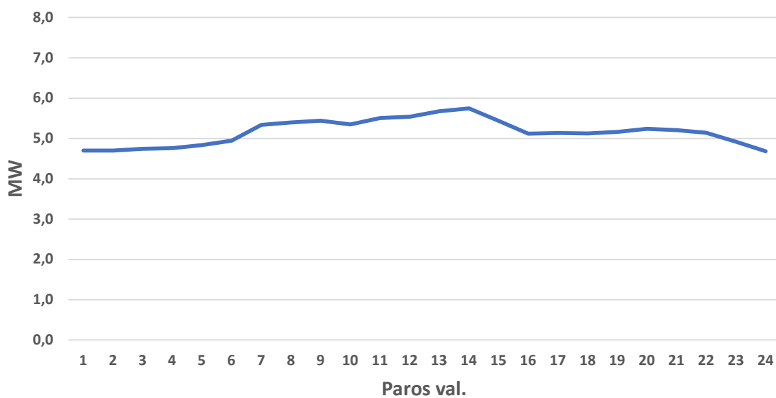
Paros vidutinis šilumos poreikio grafikas šildymo sezono metu Pasvalyje
