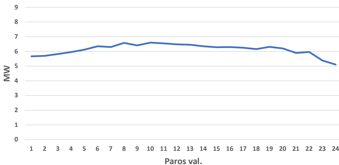
Paros vidutinis šilumos poreikio grafikas šildymo sezono metu Kupiškyje
