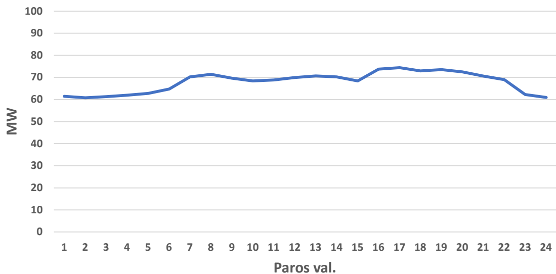
Paros vidutinis šilumos poreikio grafikas šildymo sezono metu Panevėžyje
