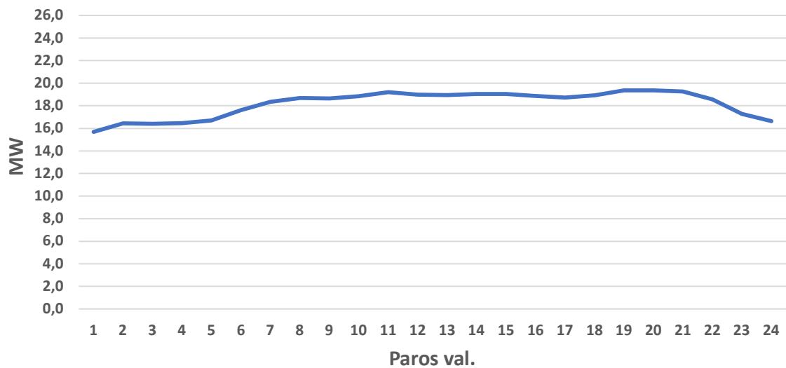
Paros vidutinis šilumos poreikio grafikas šildymo sezono metu Kėdainiuose
